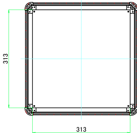
C-C ( 1 : 6 )
