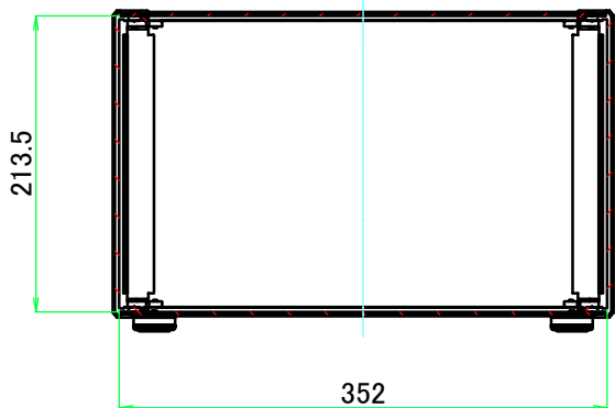
A-A ( 1 : 6 )
